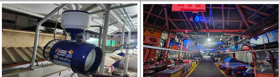
증발냉방장치
